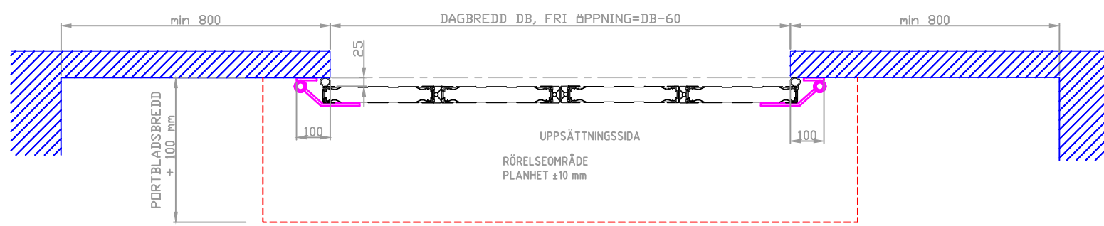
A-A HORIZONTALSEKTION
