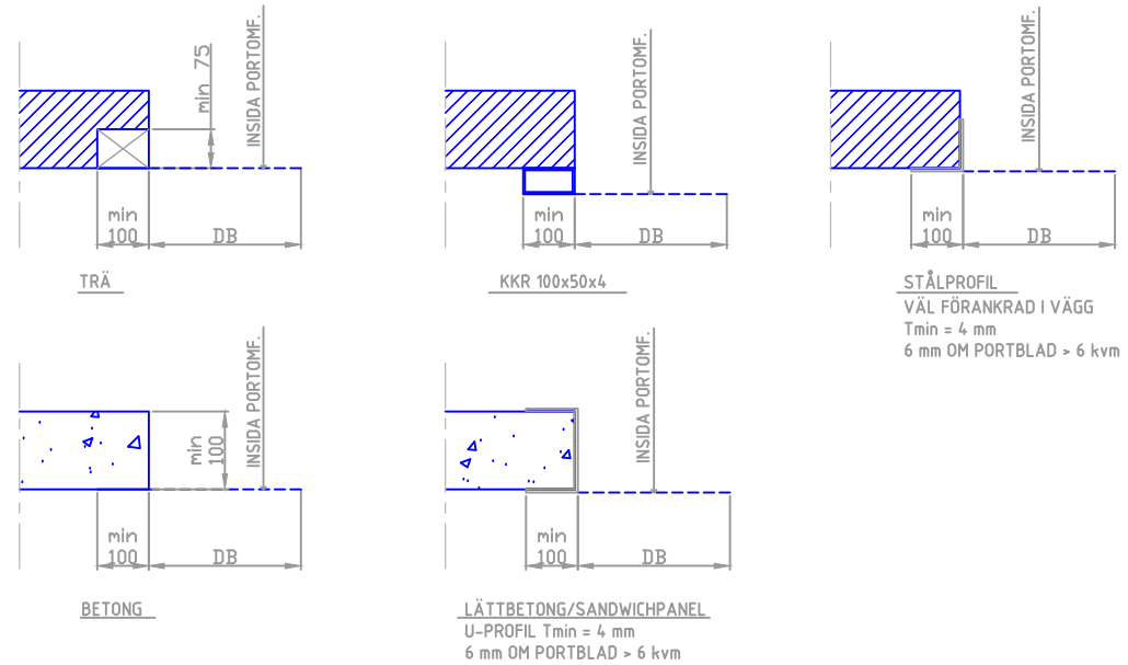
ALT. STÄNDARE
