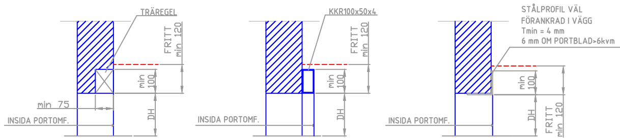
ALT. ÖVERLIGGARE
