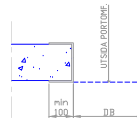
LÄTTBETONG/SANDWICHPANEL U-PROFIL T min = 4 mm 6 mm OM PORTBLAD > 6 kvm
