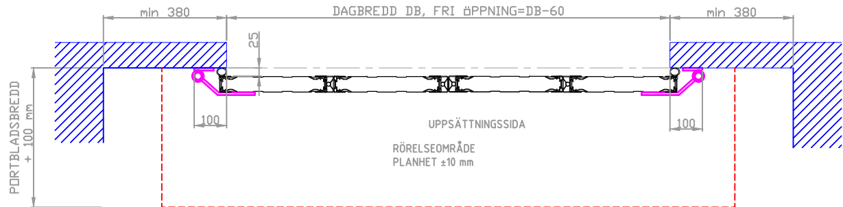
A-A HORIZONTALSEKTION
