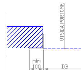
STÅLPROFIL VÅL FÖRANKRAD I VÄGG T min = 4 mm 6 mm OM PORTBLAD > 6 kvm
