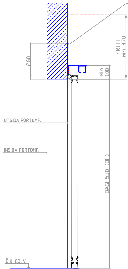
VERTIKALSEKTION
