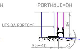
TÄTNING MOT GOLV
