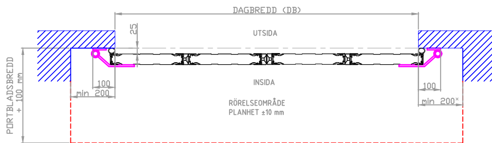
A-A HORIZONTALSEKTION
